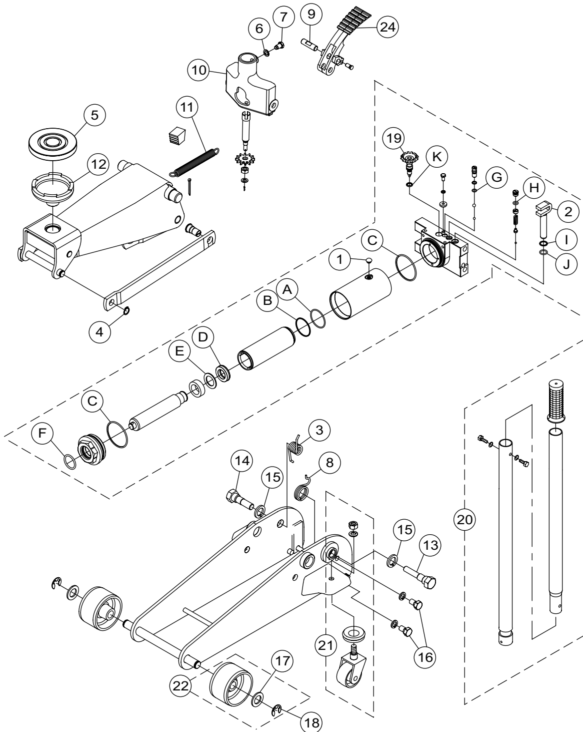
Figure 3 : Illustration des pièces de rechange du modèle 21030B
