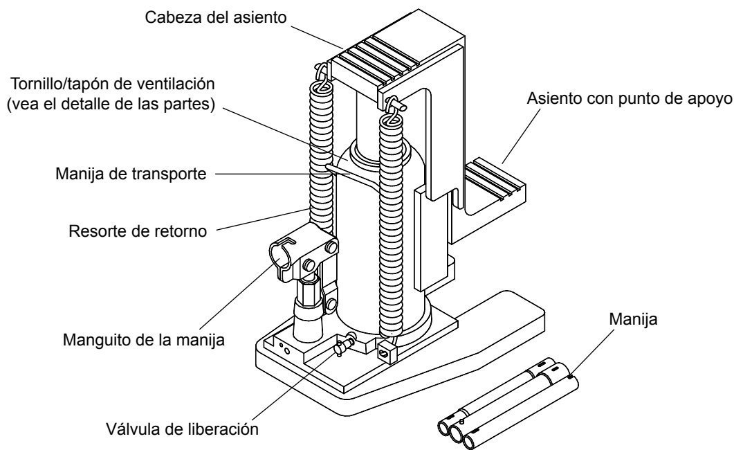
Figura 1: Nomenclaturas 13060, 13120 y 13200
