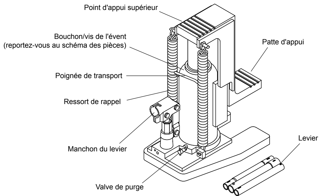
Figure 1 - Pièces des modèles 13060, 13120 et 13200
