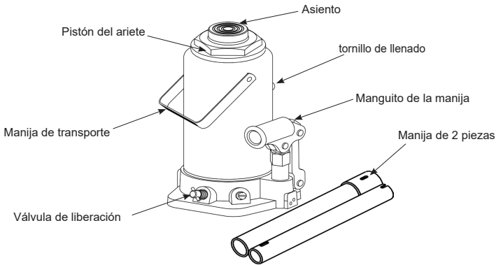
Figura 1: Nomenclatura habitual de un gato de botella
