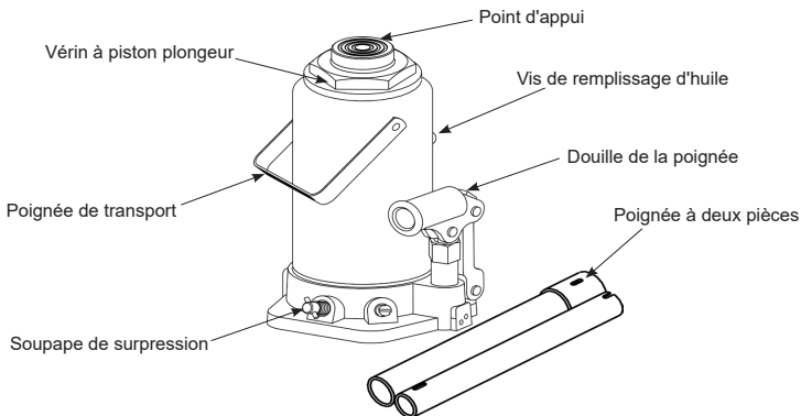
Figure 1 : Pièces d'un cric-bouteille typique
