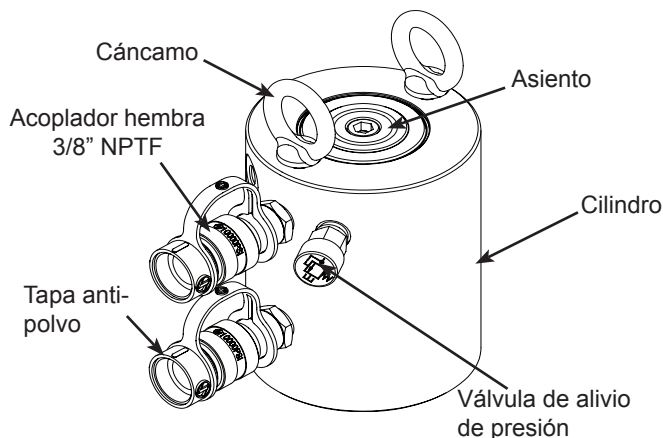
Figura 1: Componentes habituales del cilindro
