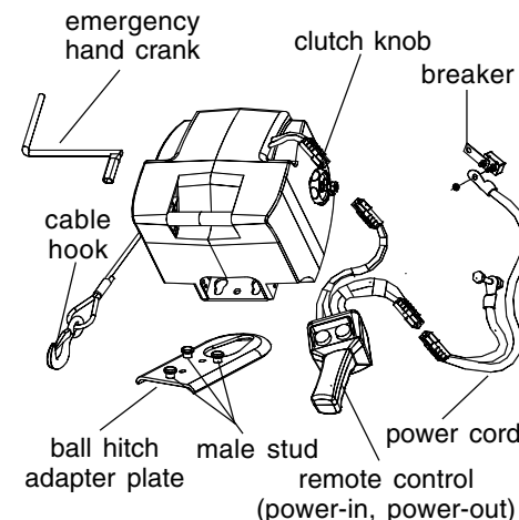
Fig. 2 - P-1100 Nomenclature
