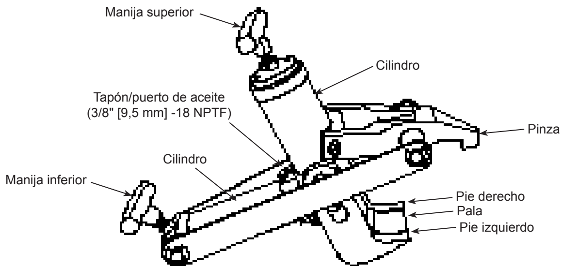
Figura 1: Componentes del modelo J22910
