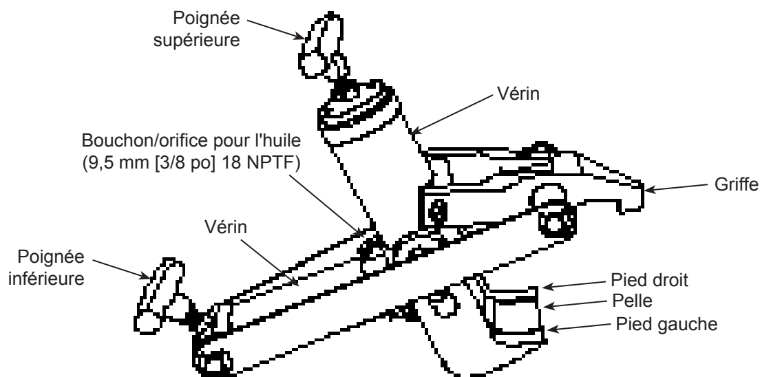
Figure 1 : Composants du modèle J22910
